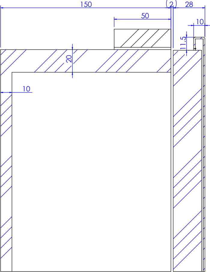
局部视图 AH 比例 1 : 2
