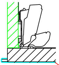
DETALLE C
