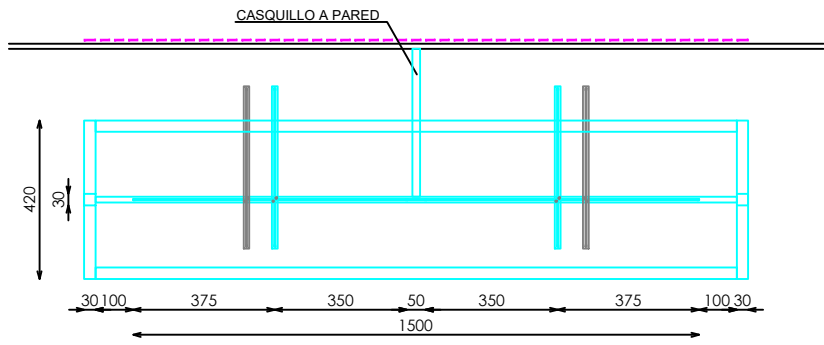
PLANTA
