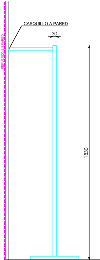
ALZADO LATERAL
