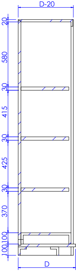
剖面 AG-AG
