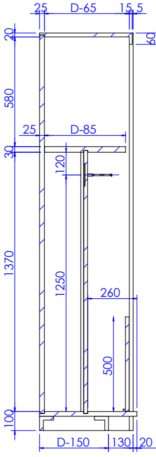
剖面 AH-AH
