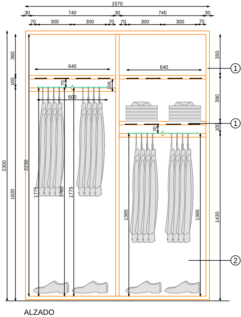
ALZADO
