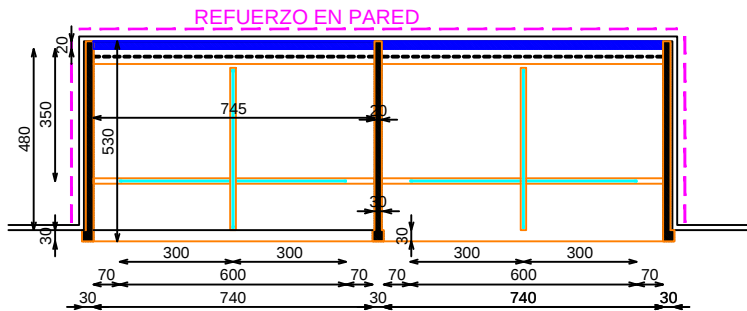
PLANTA
