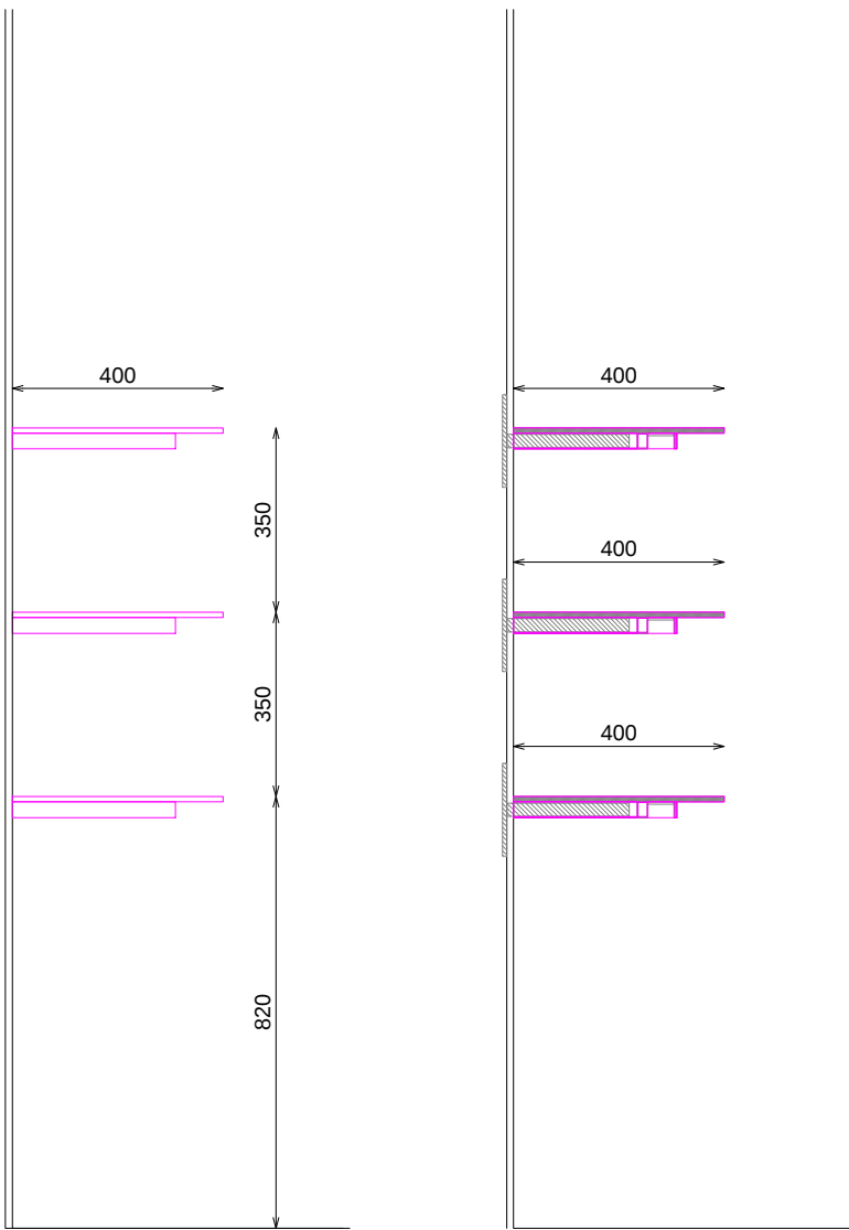
PERFIL
