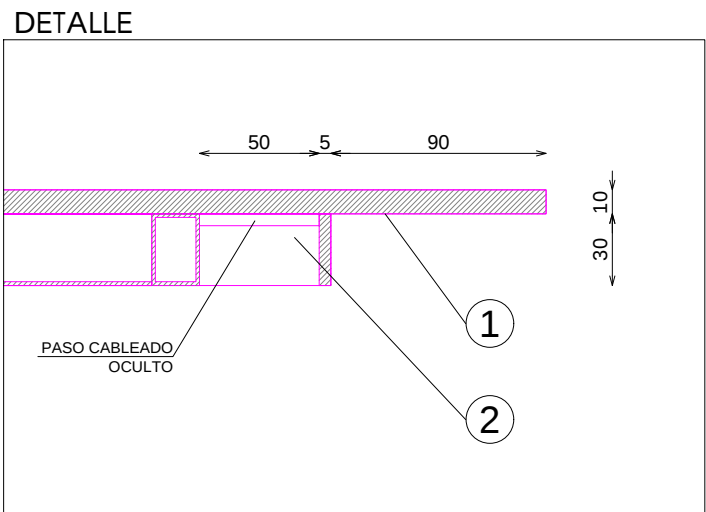
DETALLE
