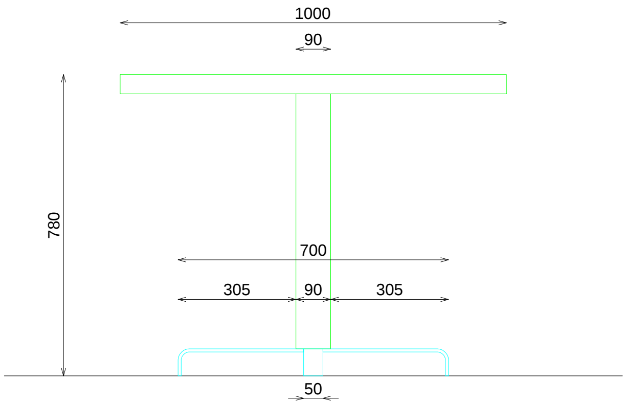
ALZADO LATERAL
