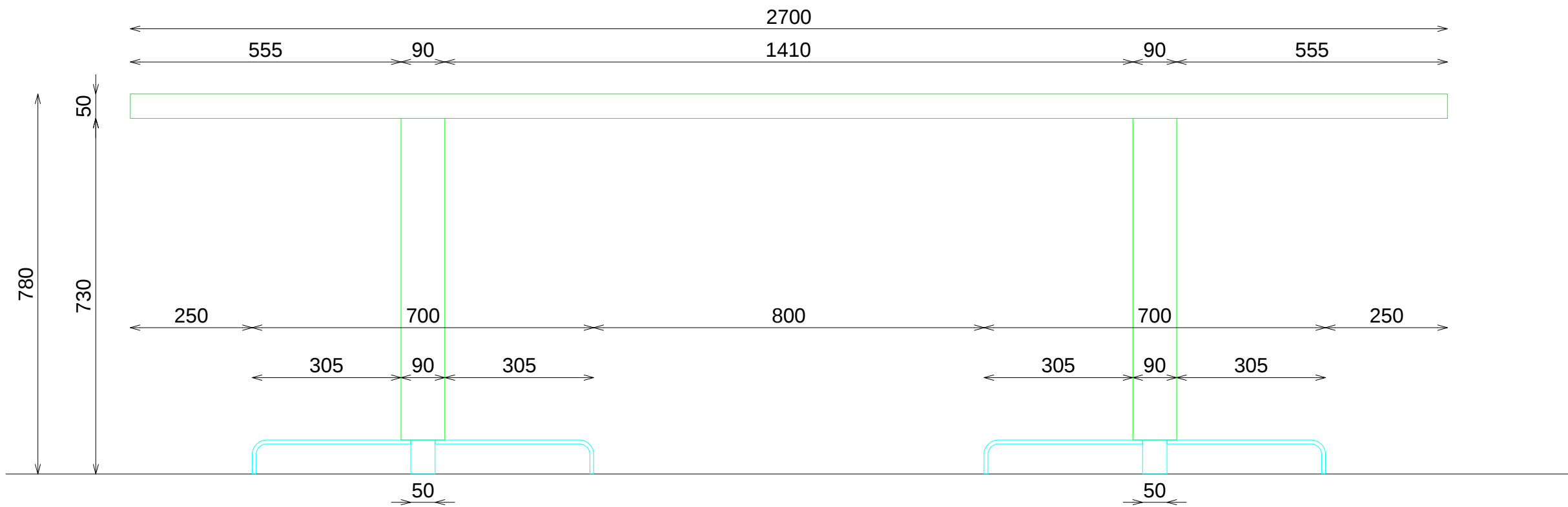
ALZADO FRONTAL
