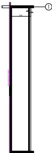
SECCIÓN PANEL
