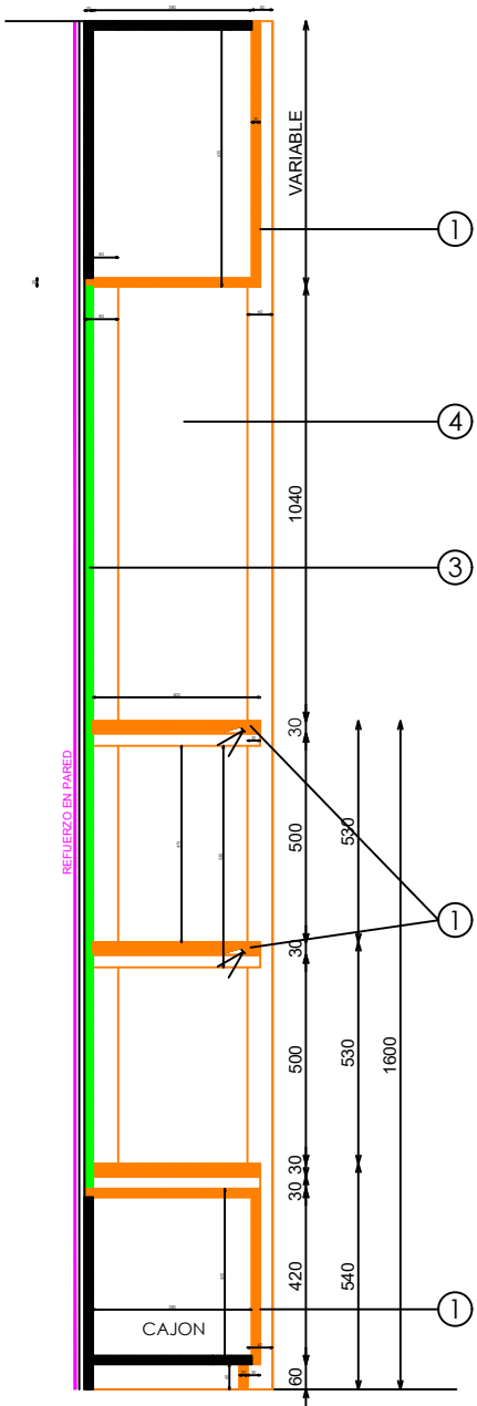
SECCION
