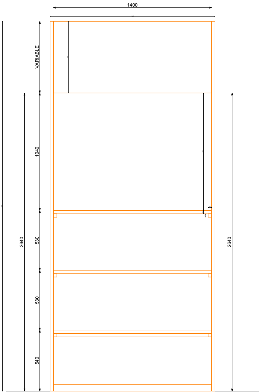
ALZADO
