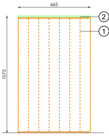
ALZADO LATERAL
