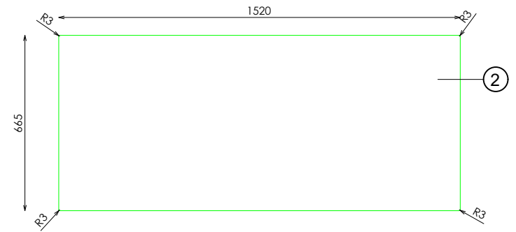
PLANTA
