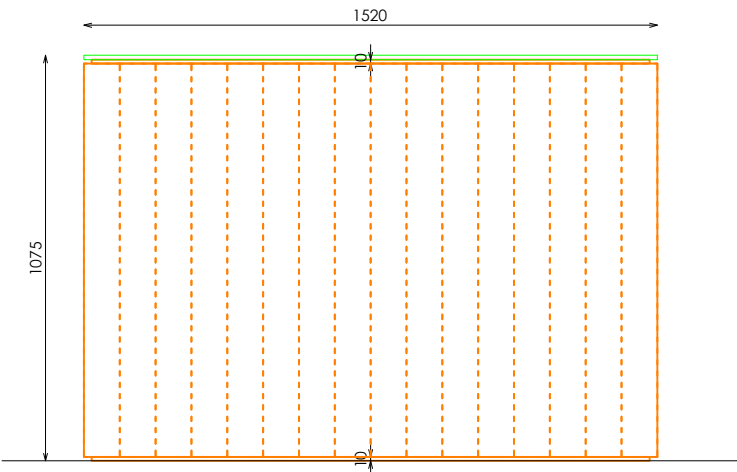
ALZADO FRONTAL
