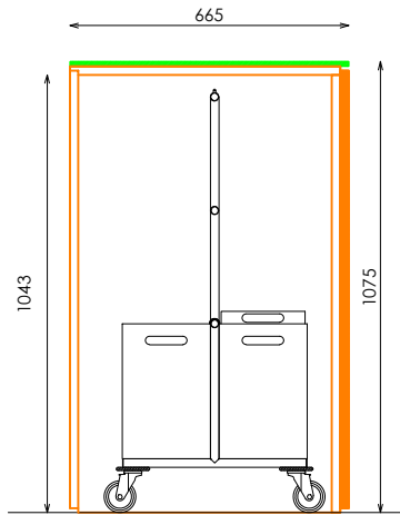
SECCION
