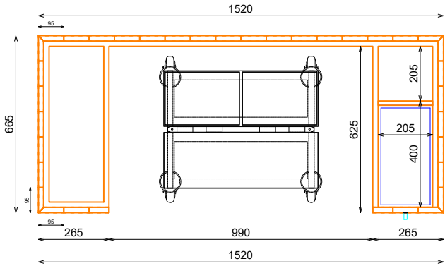
PLANTA SECCIONADA
