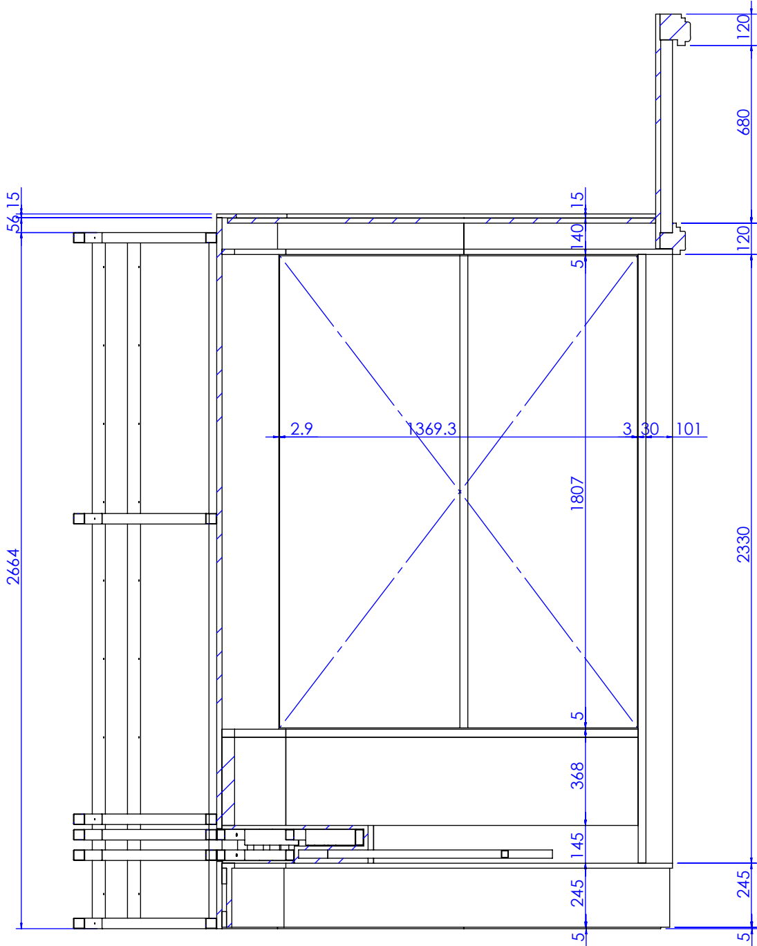
剖面 B-B
