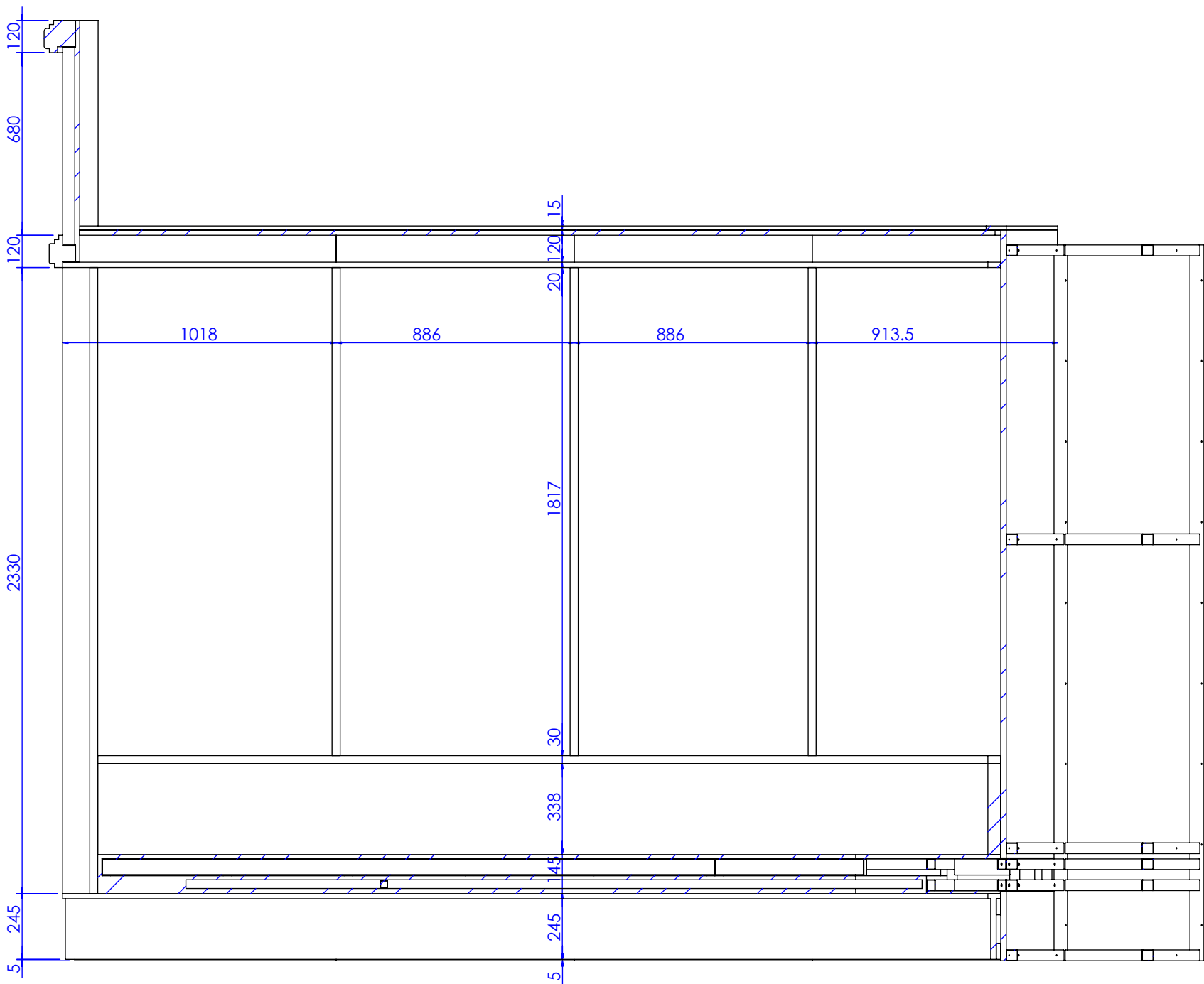
剖面 C-C
