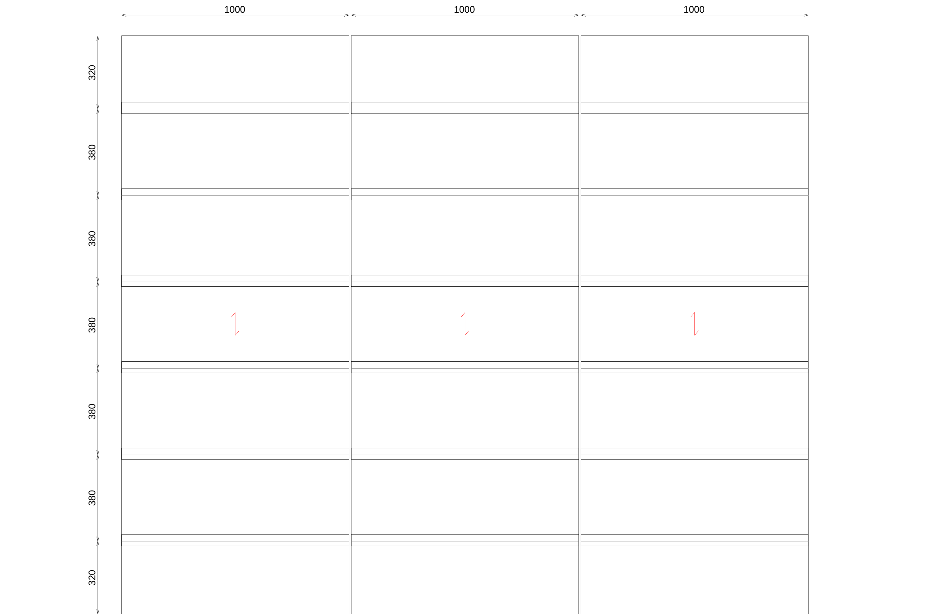
ALZADO
