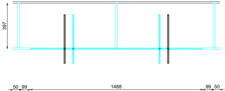
ALZADO FRONTAL
