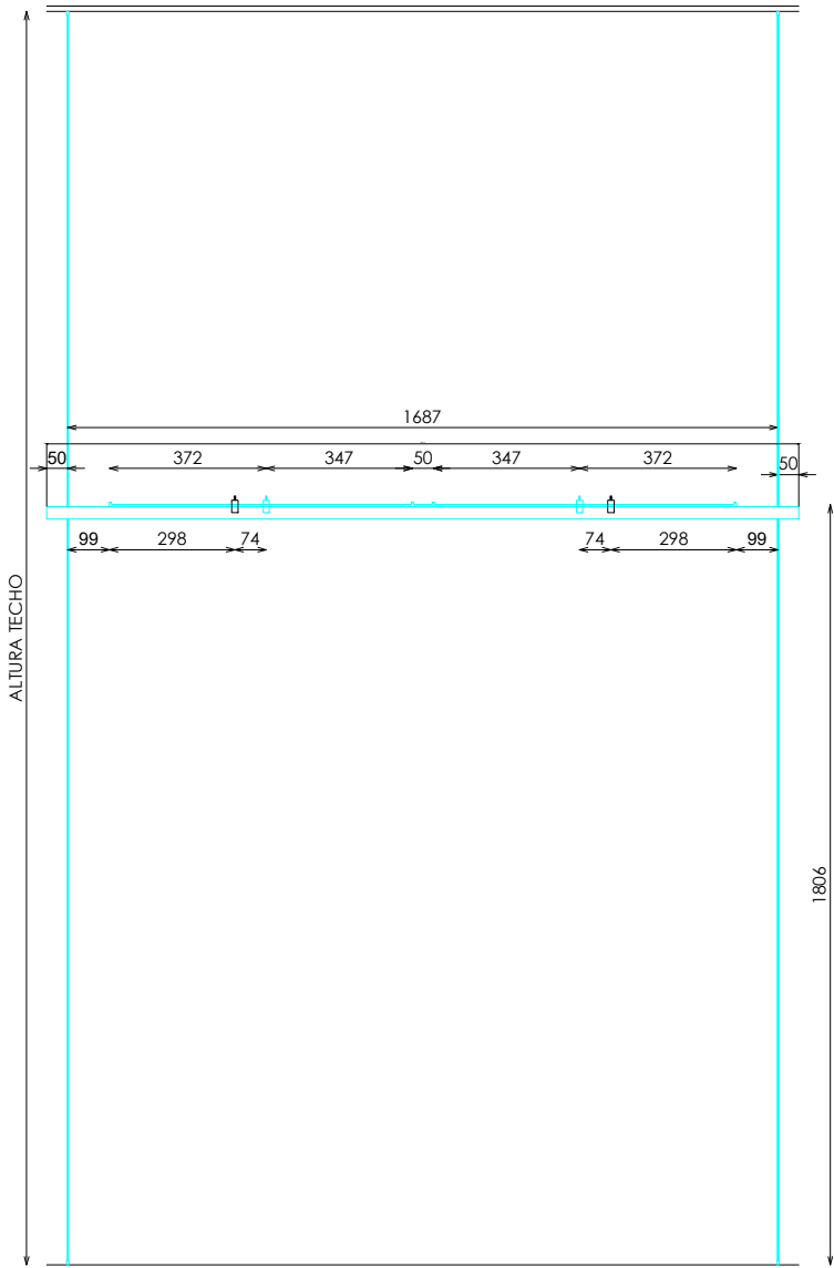
ALZADO FRONTAL
