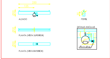
DETALLE FRONTALES EXTRAIBLES
