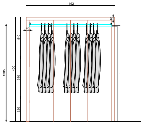
ALZADO
