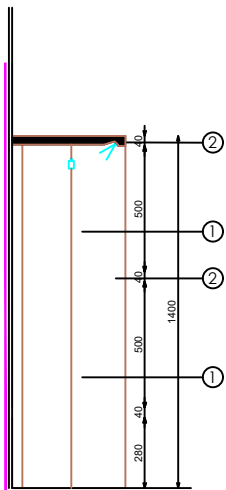
SECCION
