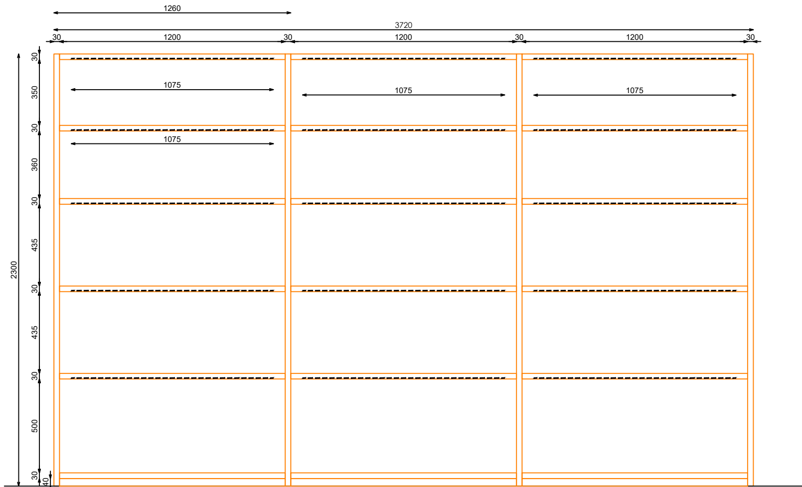
ALZADO
