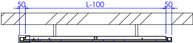
剖面 AI-AI
