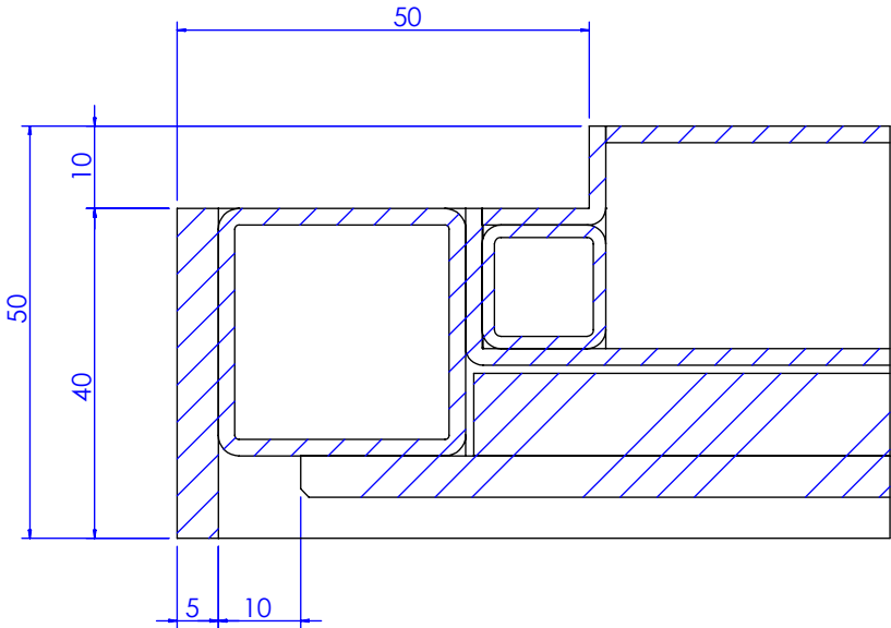
局部视图 AJ 比例 1 : 1
