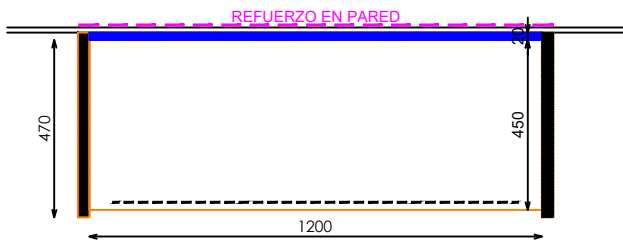
PLANTA SECCIONADA
