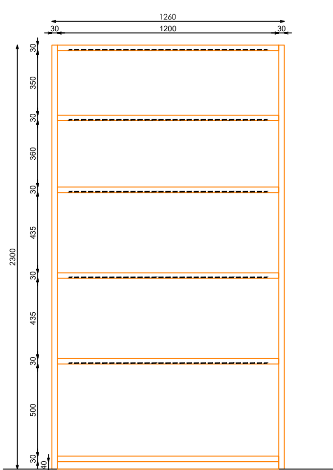
ALZADO
