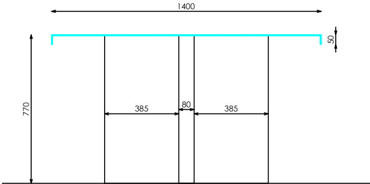
ALZADO LATERAL
