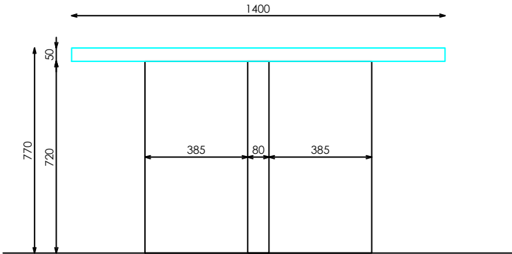
ALZADO FRONTAL
