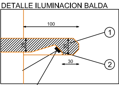
SECCION
