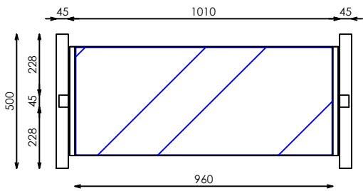
PLANTA
