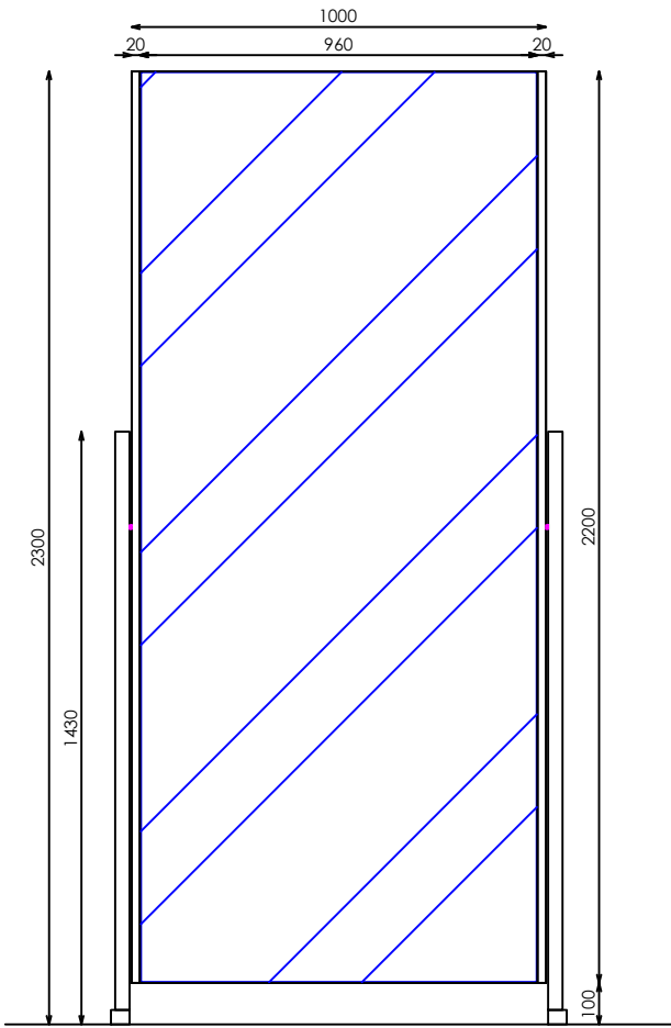
ALZADO FRONTAL
