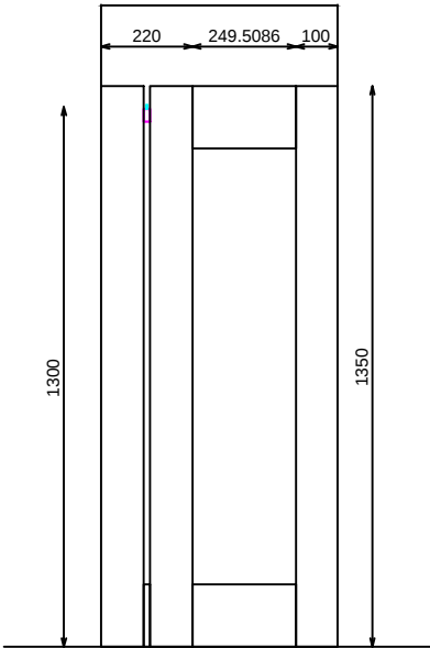
ALZADO DERECHO
