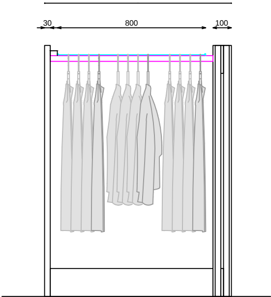
ALZADO
