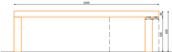
ALZADO FRONTAL
