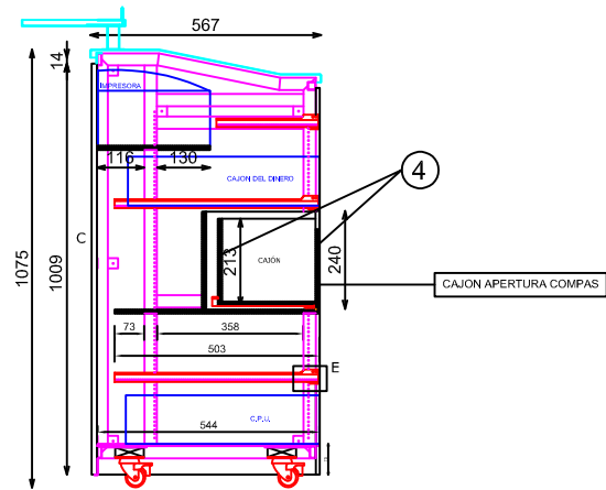
SECCIÓN
