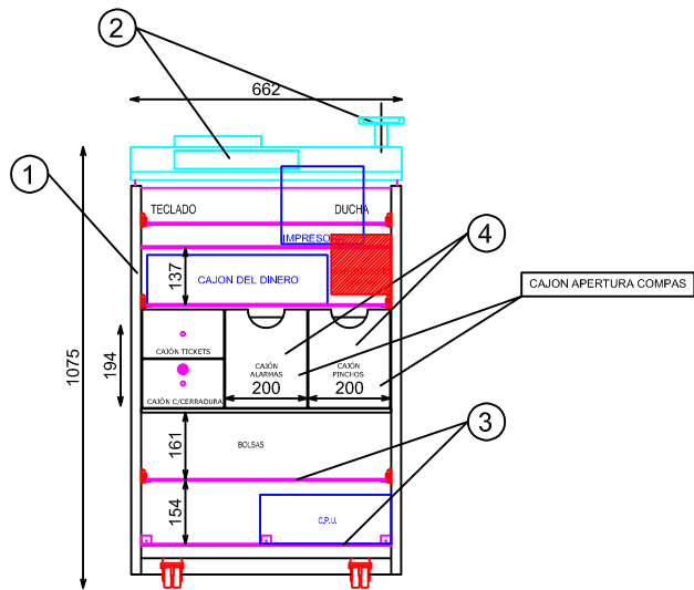
ALZADO
