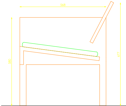
SECCIÓN
