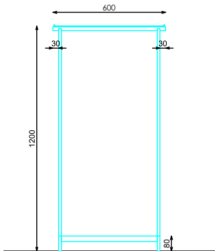
ALZADO
