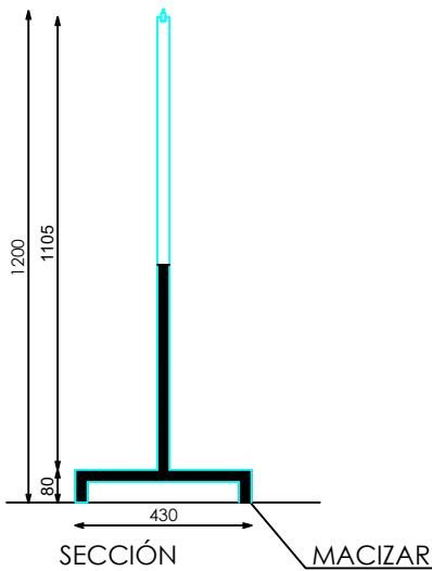
SECCIÓN
