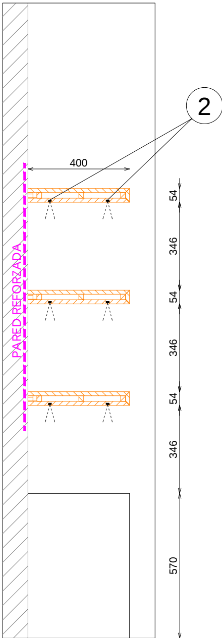
SECCIÓN
