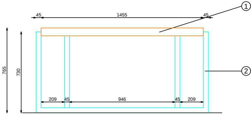
ALZADO LATERAL
