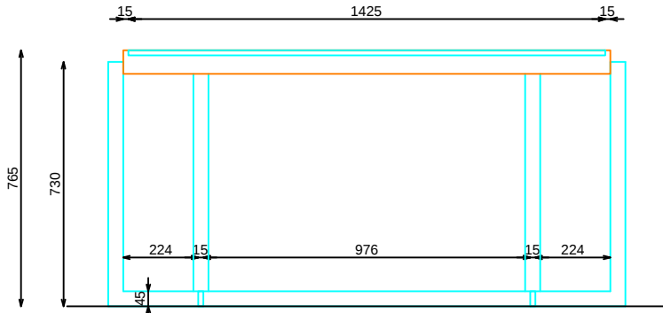
SECCION
