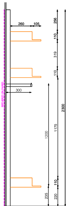
PERFIL MODULO BAS
