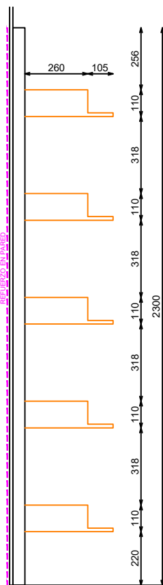
PERFIL MODULO PQ
