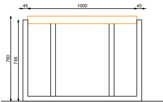
ALZADO LATERAL
