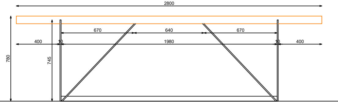
ALZADO FRONTAL
