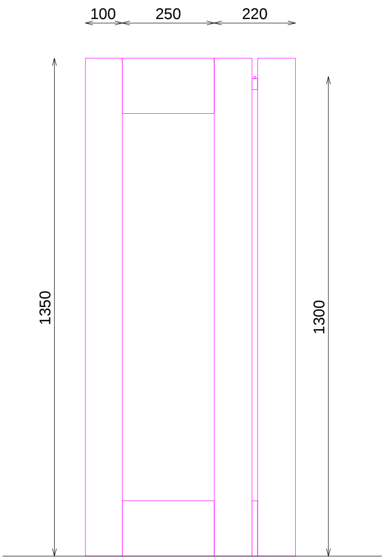
ALZADO IZQUIERDO
