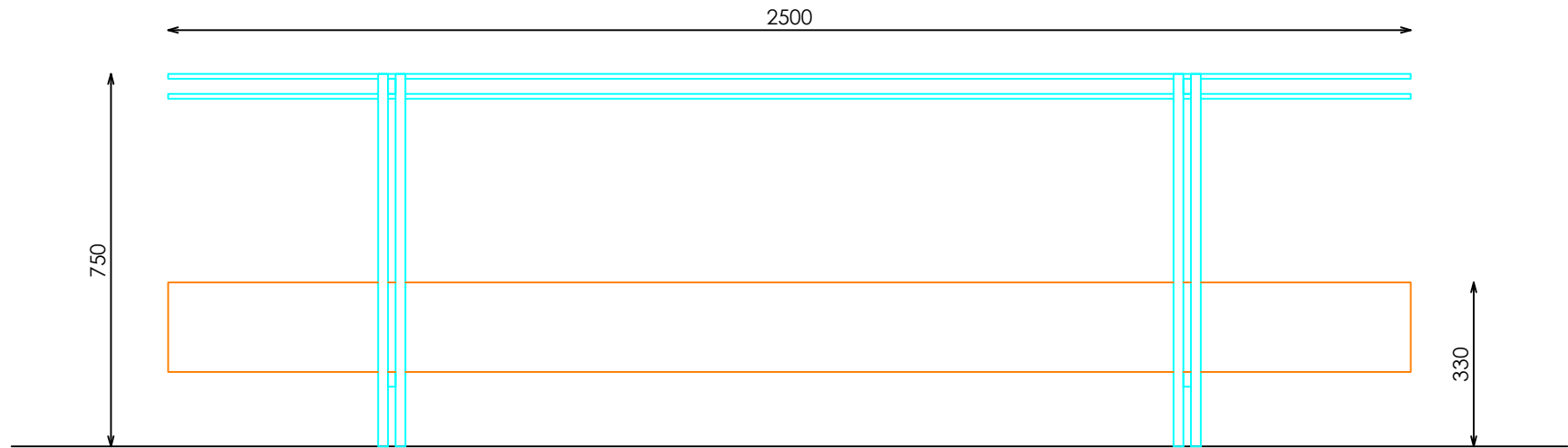
ALZADO
