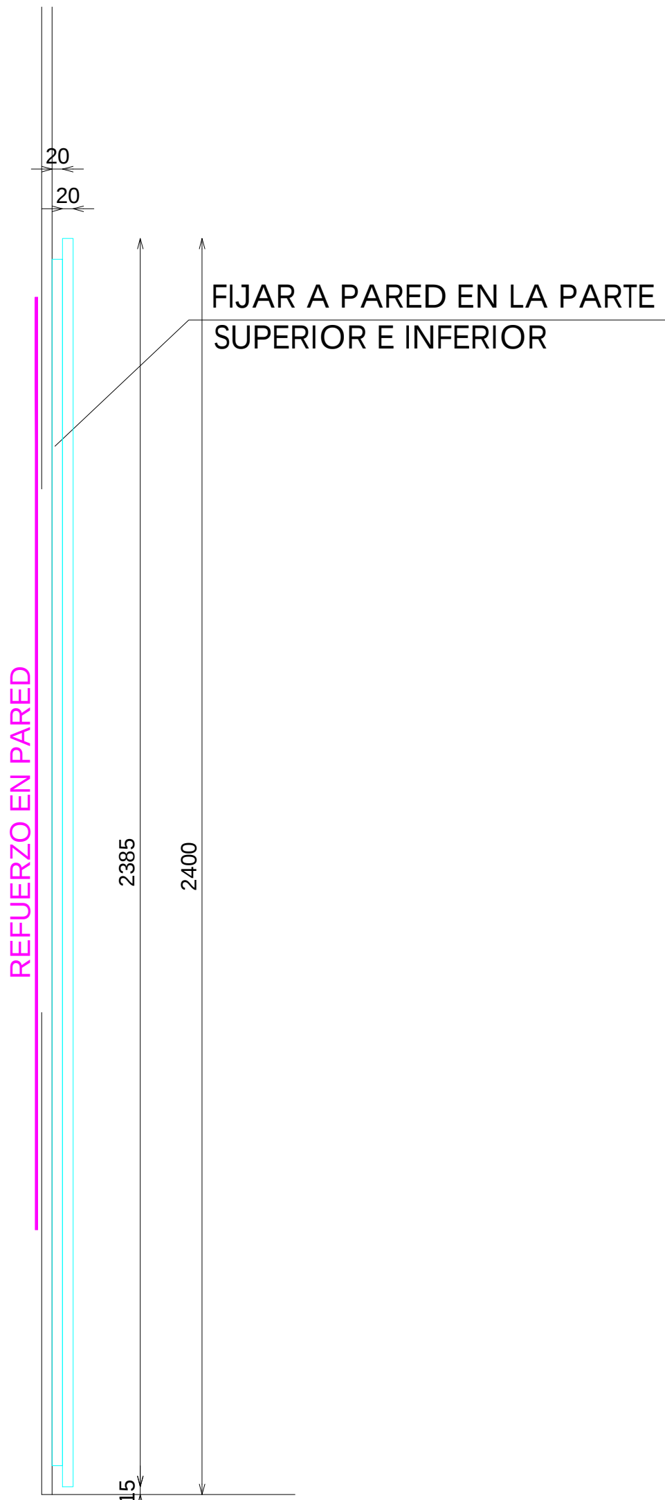
PERFIL
