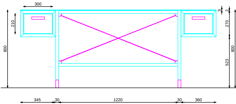
ALZADO FRONTAL
