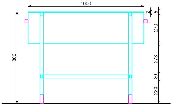
SECCION
