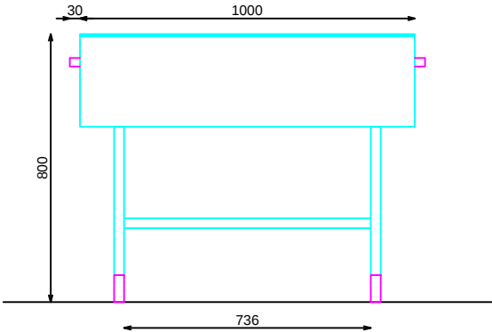
ALZADO LATERAL
