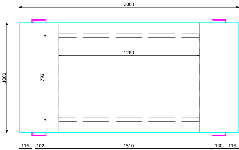
PLANTA
