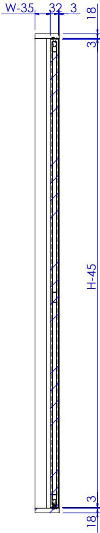
剖面 AH-AH'
