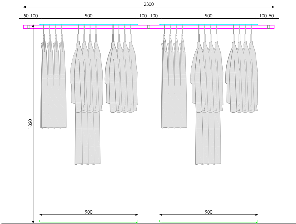
ALZADO
