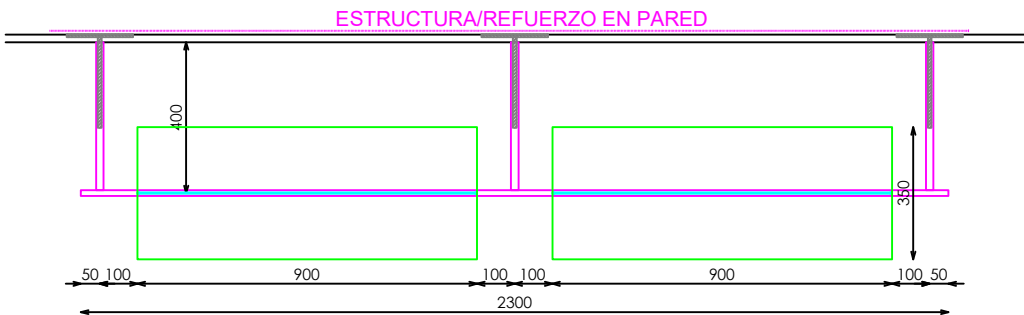
PLANTA
