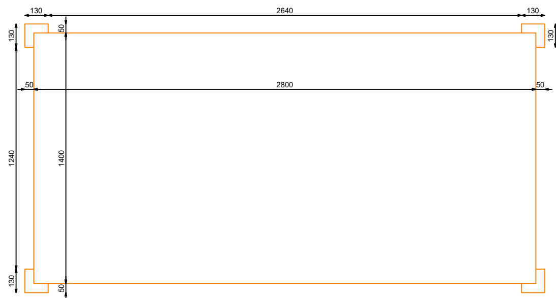
PLANTA
