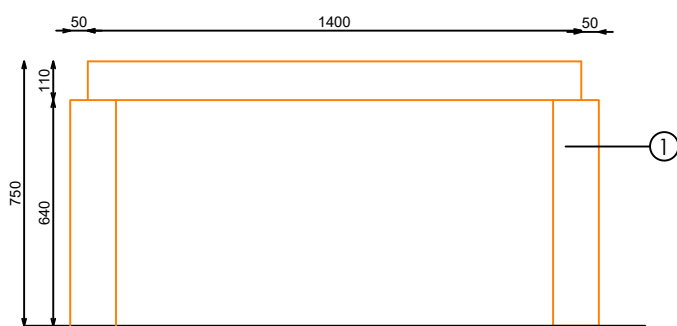
ALZADO LATERAL
