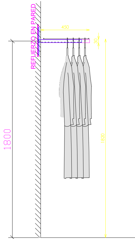
SECCION
