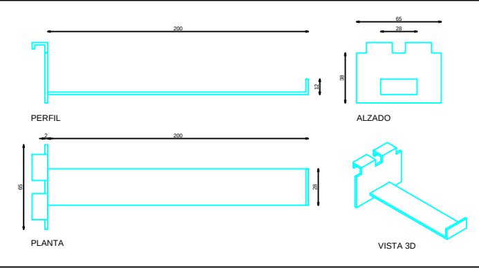
PINCHO L200
