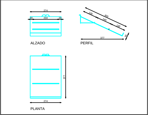
PINCHO L200
