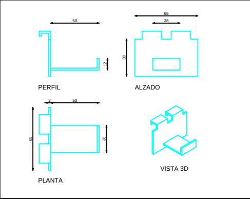
PINCHO L50
