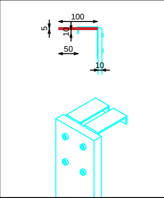
DETALLE ANCLAJE
