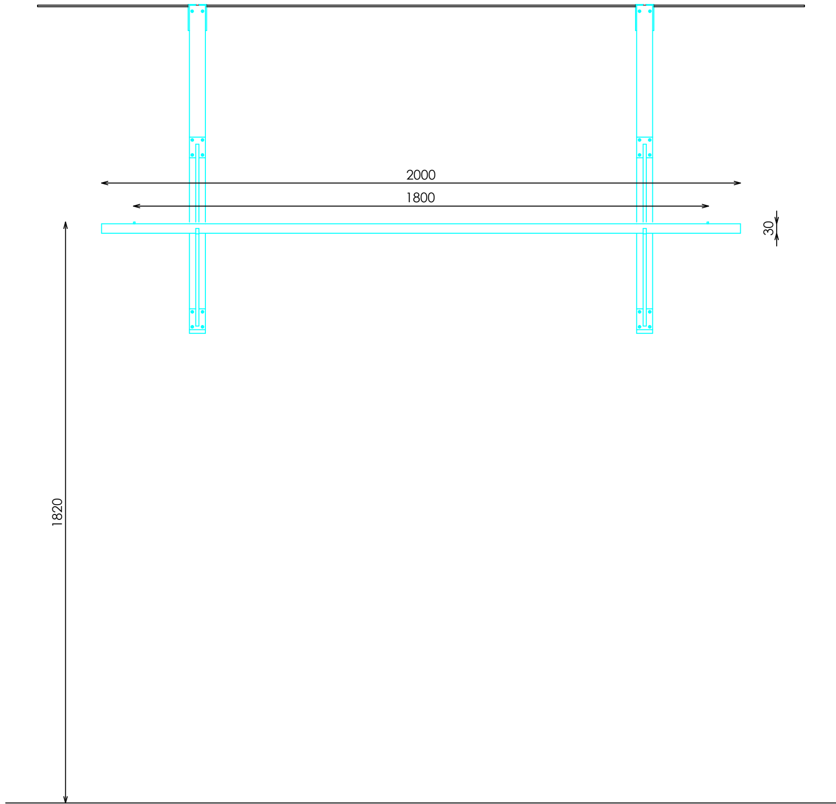
ALZADO
