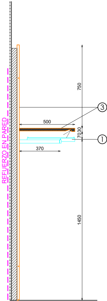
SECCION BARRA
