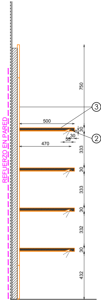
SECCION BALDAS
