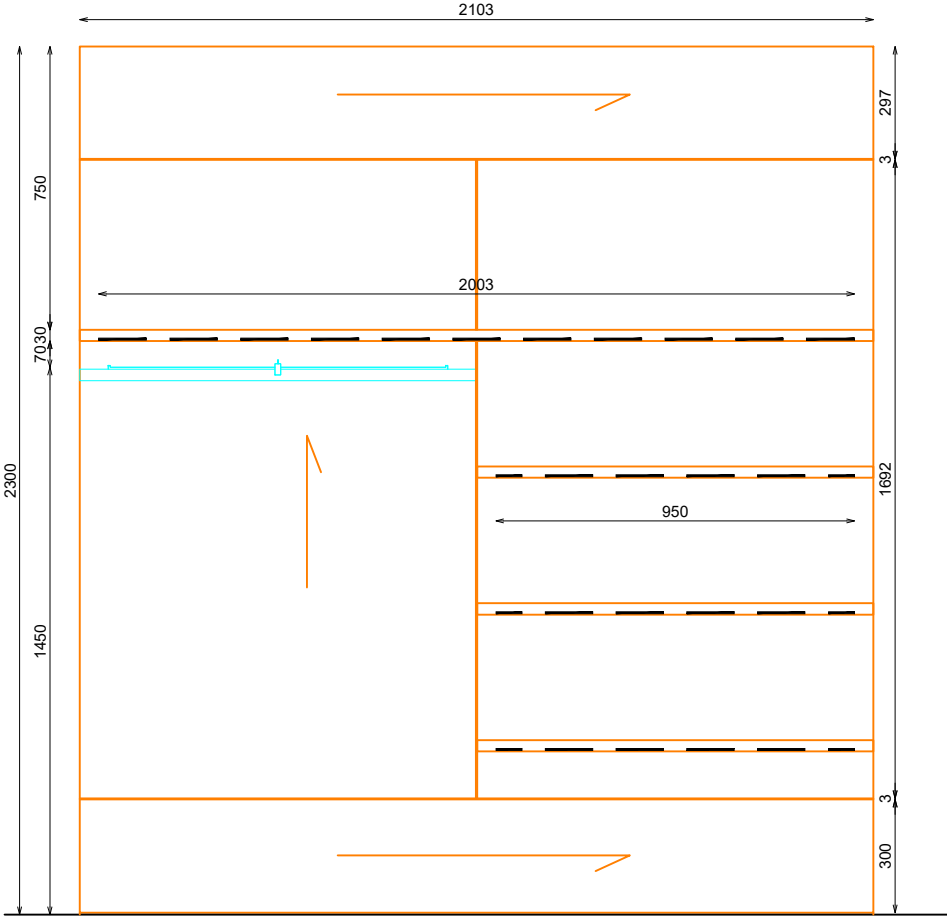
ALZADO
