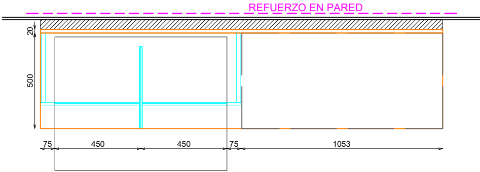
PLANTA
