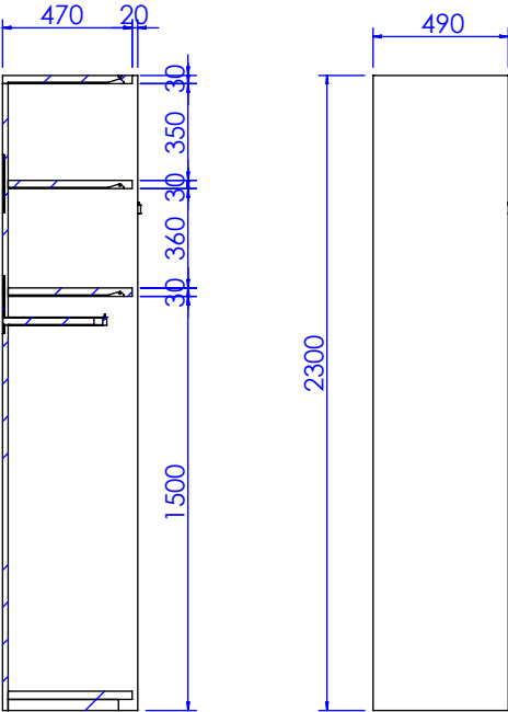
剖面 AH-AH
