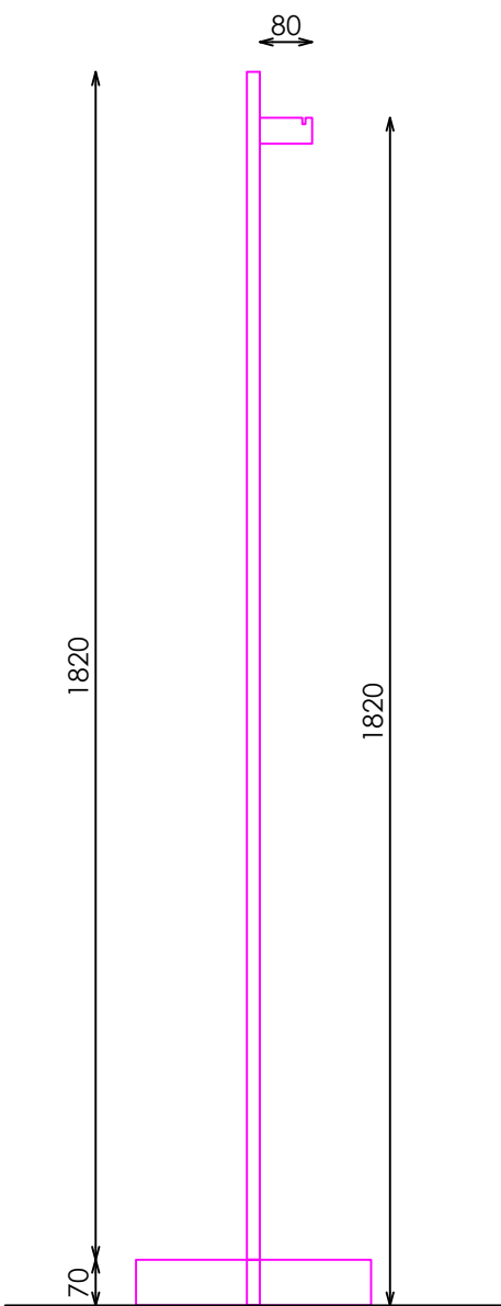
ALZADO LATERAL
