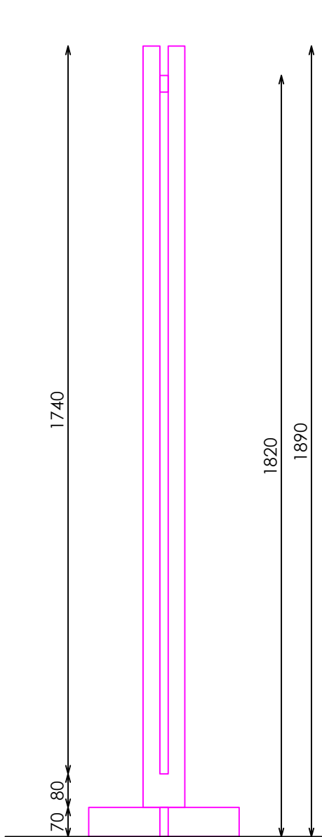
ALZADO FRONTAL
