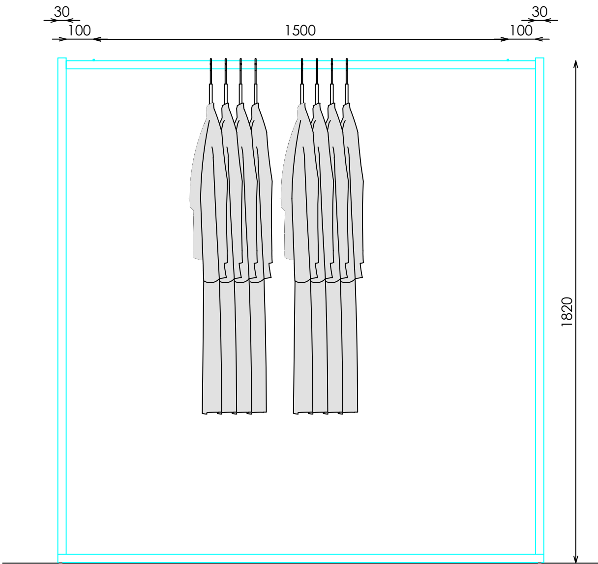
ALZADO
