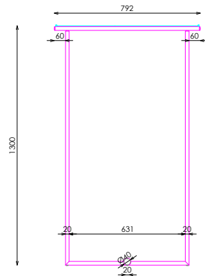
ALZADO
