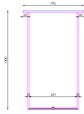
ESTRUCTURA
