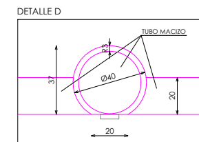
DETALLE D
