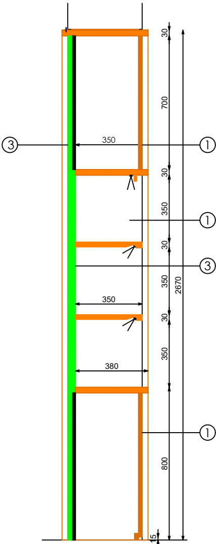
SECCION
