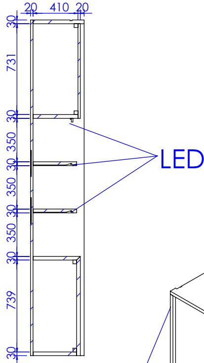
剖面 AH-AH
