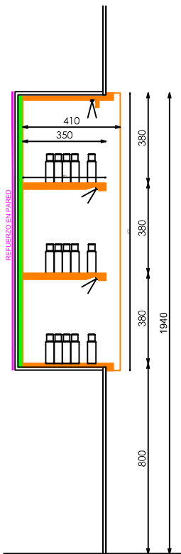
SECCION
