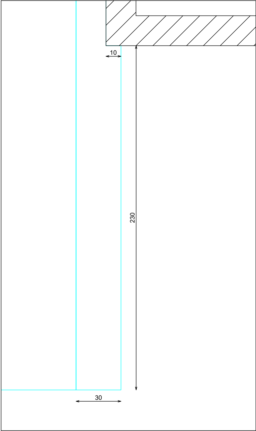
DET. LATERAL ENCUESTRO PLADUR
