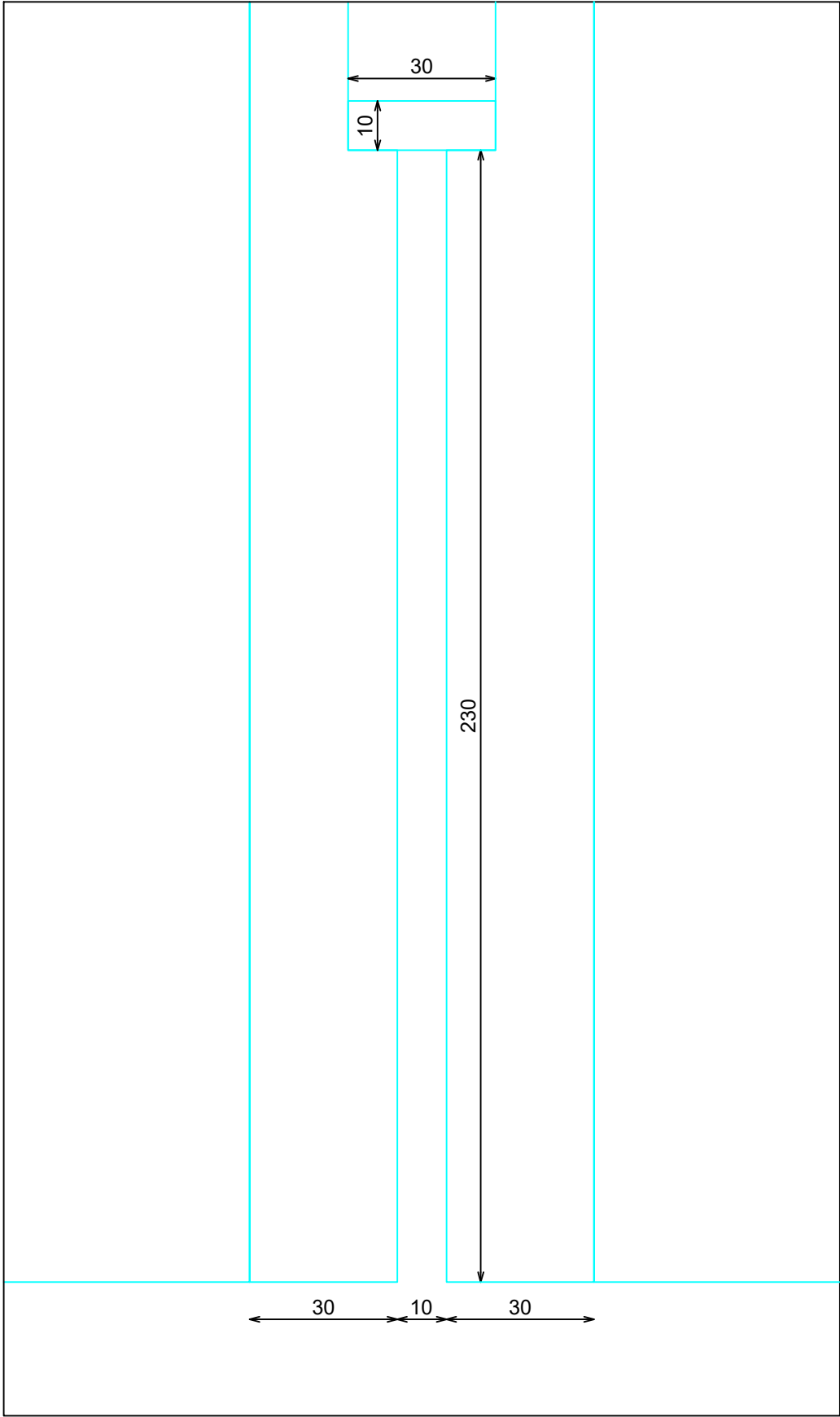
DET. LATERAL ENCUESTRO CONTINUIDAD MUEBLE
