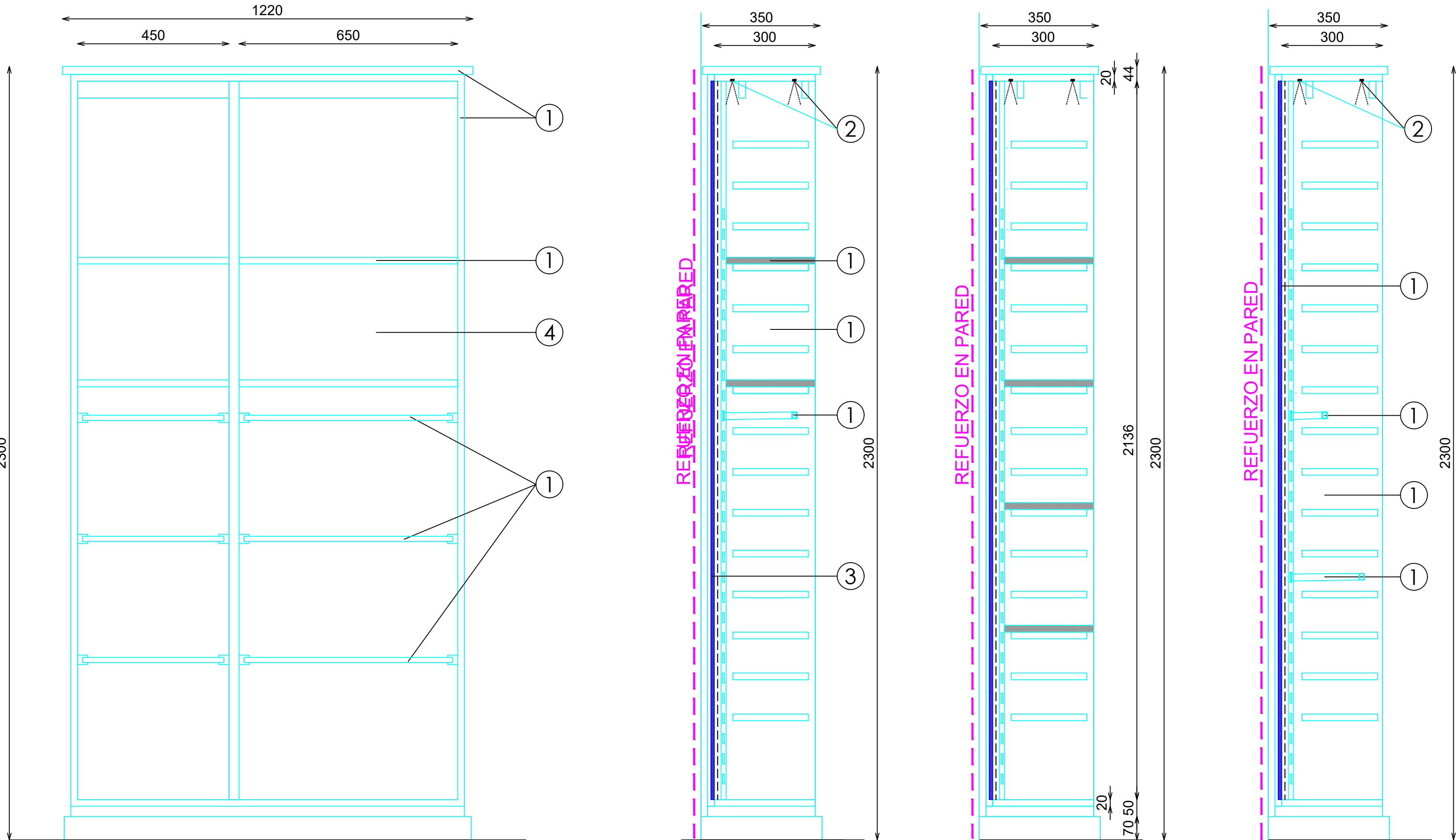
ALZADO FRONTAL ABIERTO
