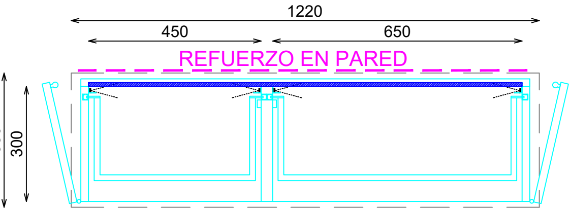
PLANTA SECCIONADA DOTACION BARRAS/PINCHOS
