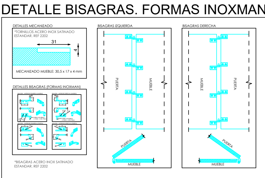
DETALLE BISAGRAS. FORMAS INOXMAN
