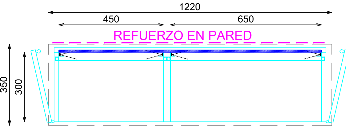
PLANTA SECCIONADA BALDAS
