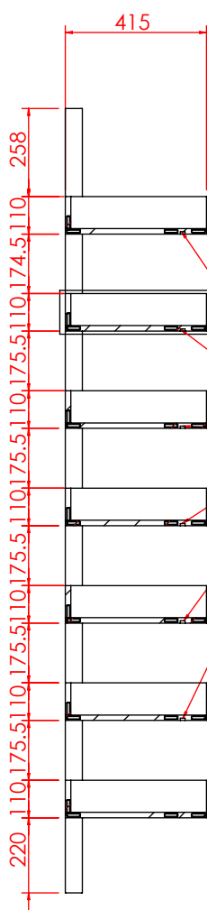
剖面 AG-AG
