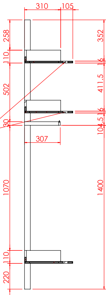
剖面 AH-AH
