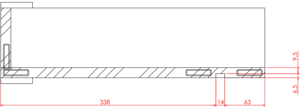
局部视图 AI 比例 1:3
