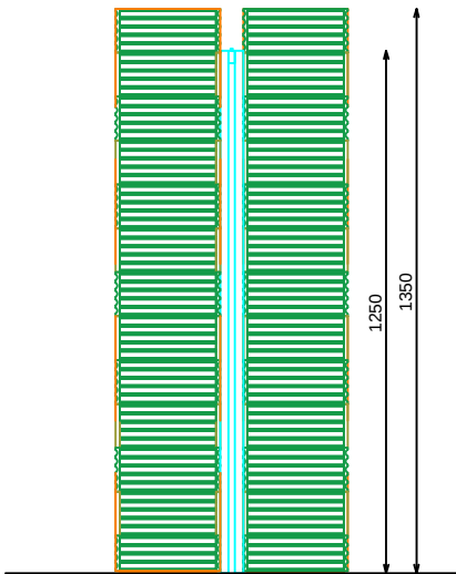
ALZADO LATERAL
